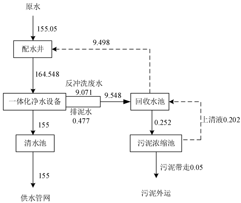
图 4-4 平安水厂水平衡图 单位: \text{m}^3/\text{d}
