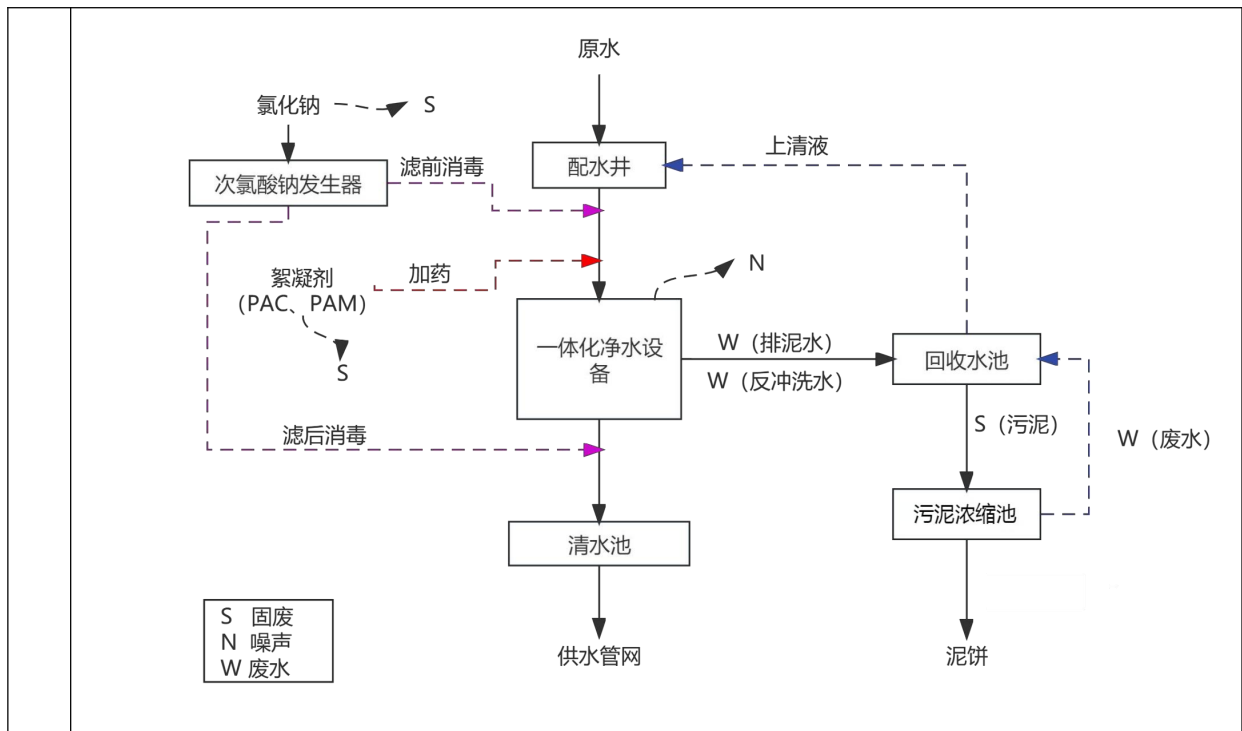
图 2-5 一体化净水厂运营期工艺流程及产污环节示意图
